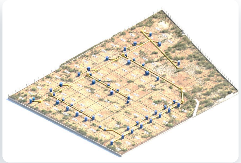
Modelación 3D del alcantarillado, Urbanización Monteverde
