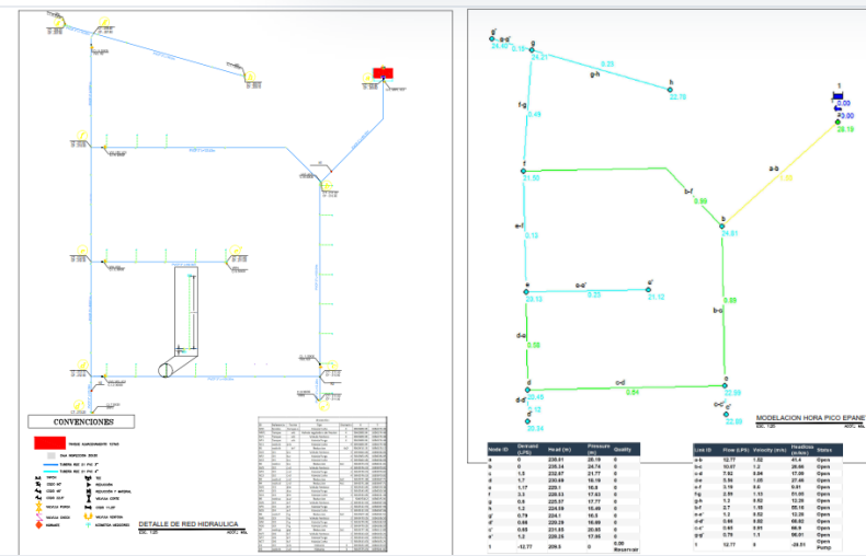
Detalle de red hidráulica y modelación en hora pico (EPANET)
