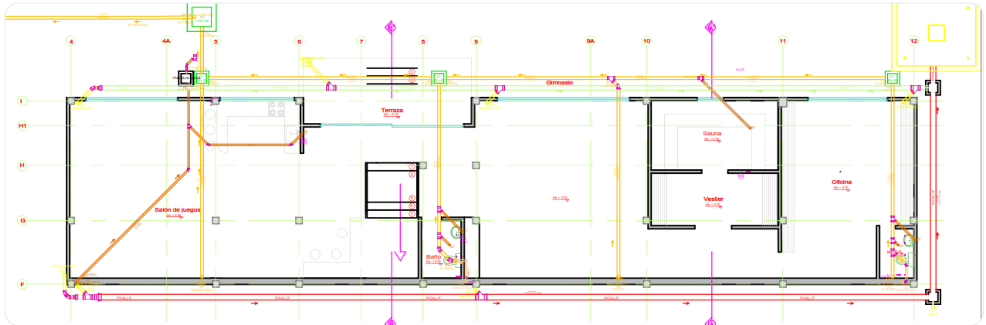
Plano de diseño de redes hidrosanitarias, proyecto Casa Yerbabuena
